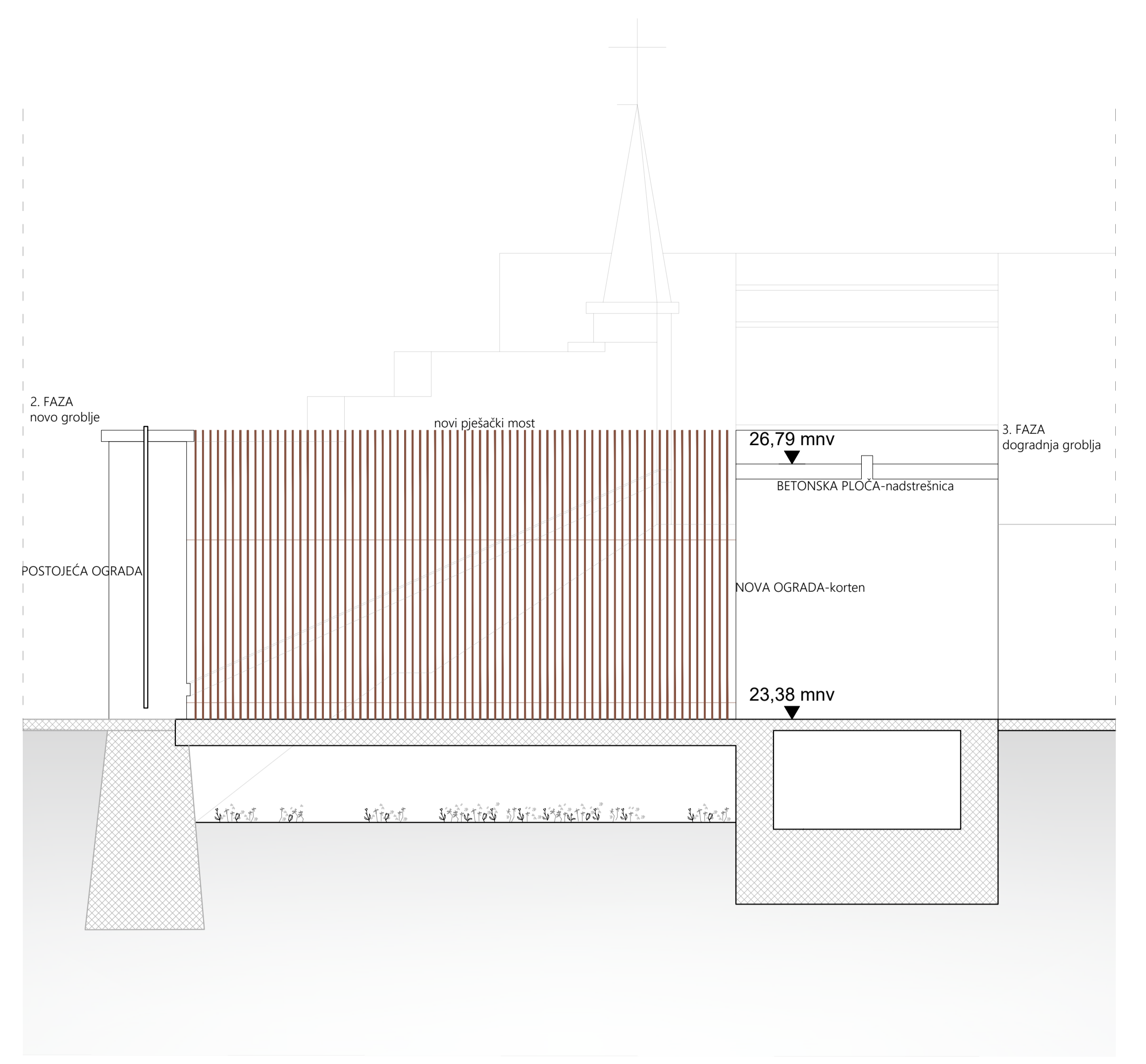
DETALJ MOSTA
