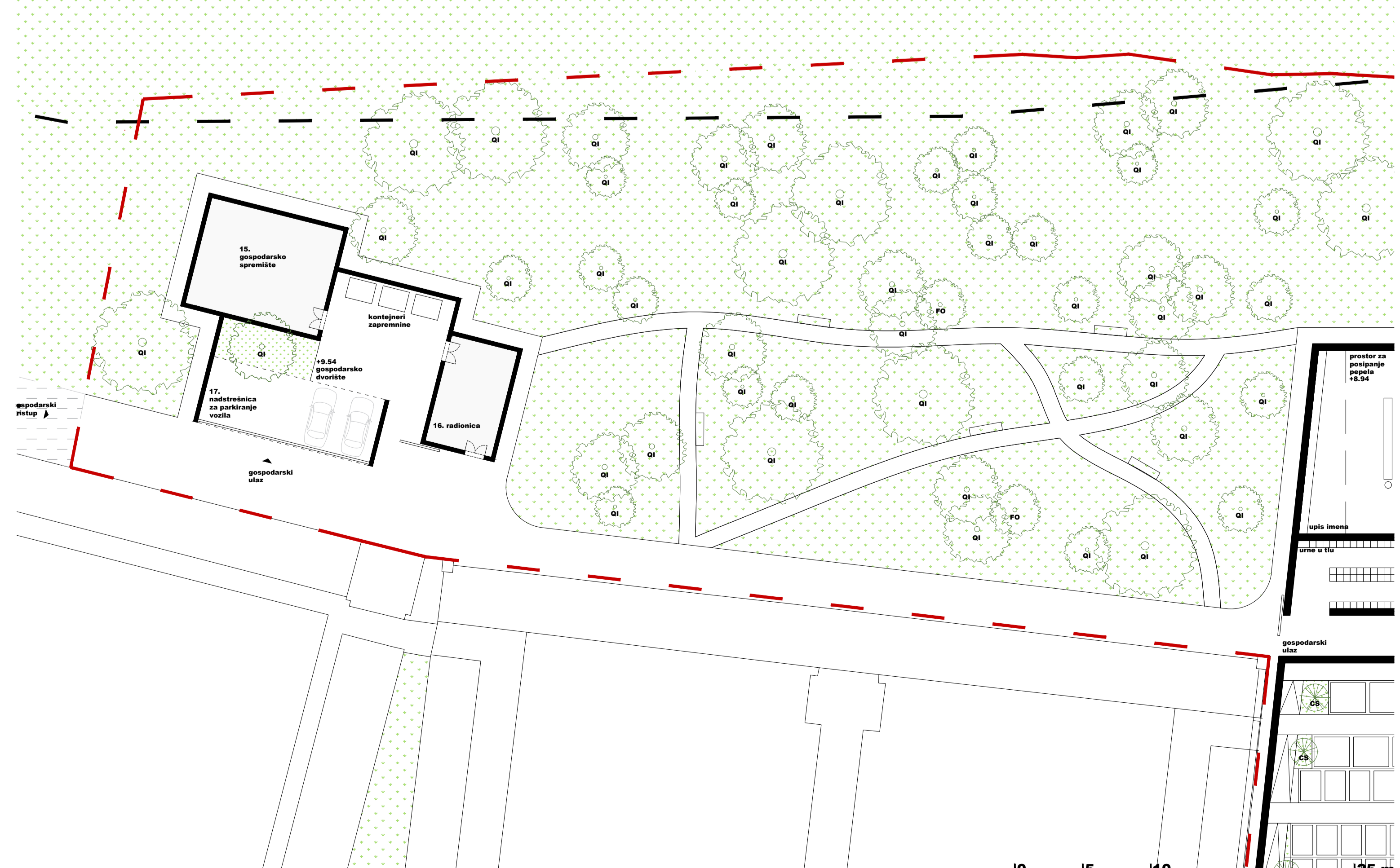
PLAN OBRADBE POVRŠINA I PRIKAZ PLANIRANE SADNJE ISJEČAK
