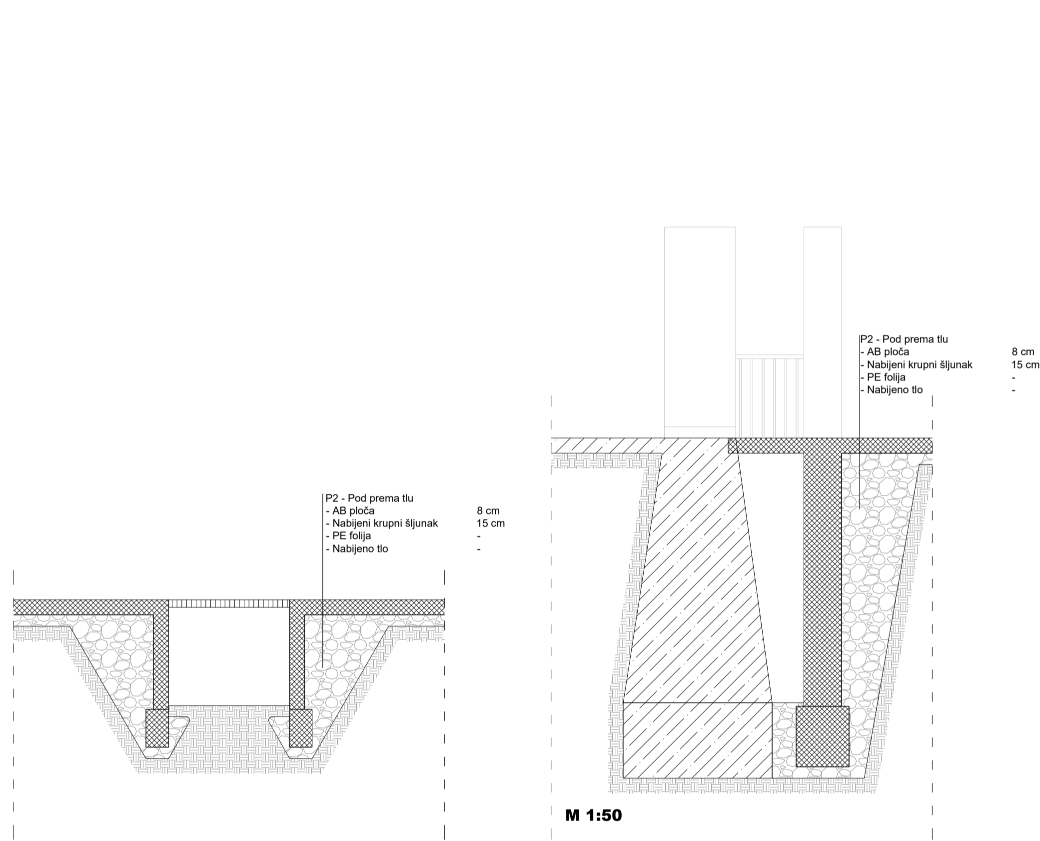
DETALJ SPOJA STAROG I NOVOG GROBLJA
