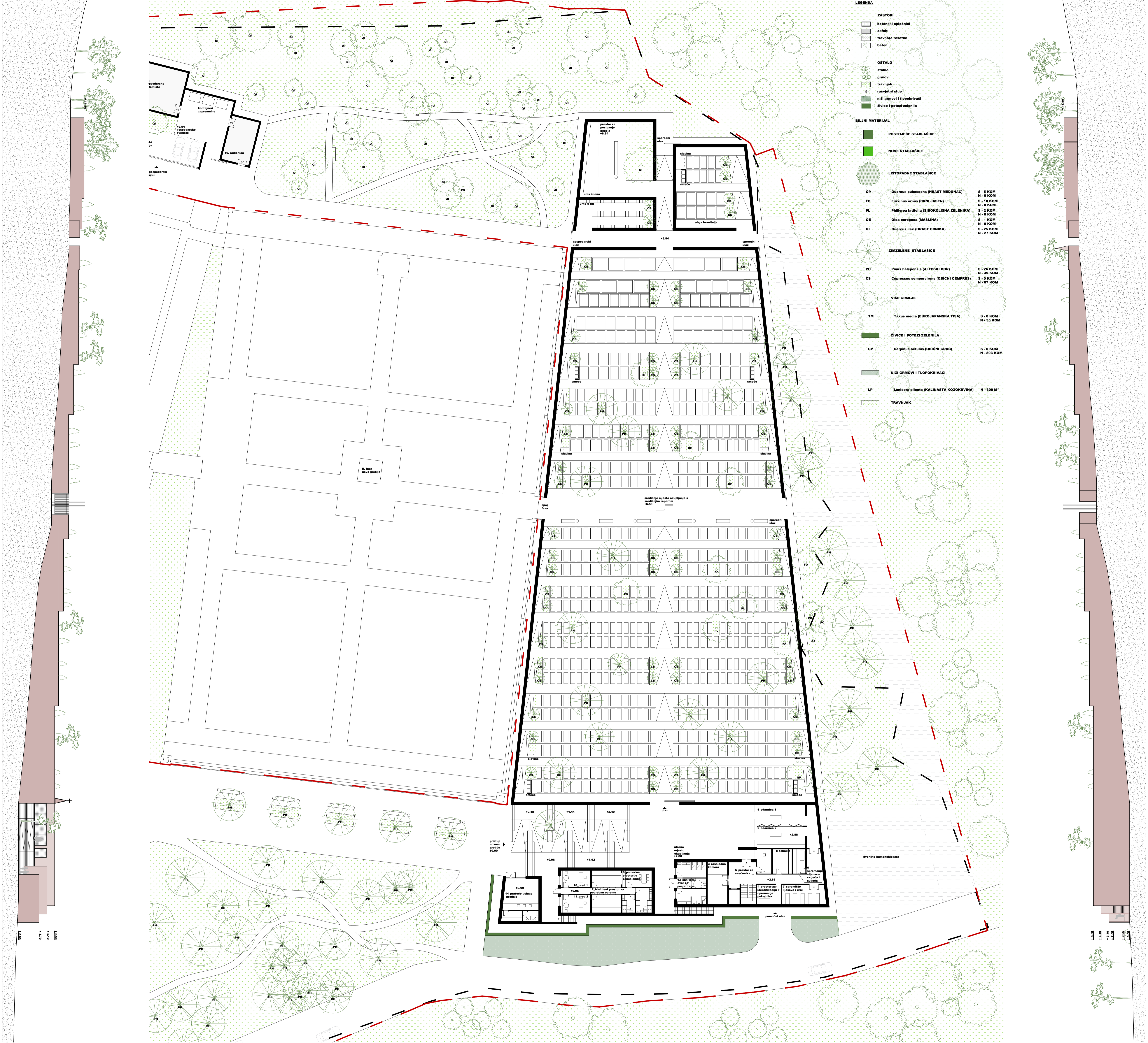
PLAN OBRADBE POVRŠINA I PRIKAZ PLANIRANE SADNJE ISJEČAK
