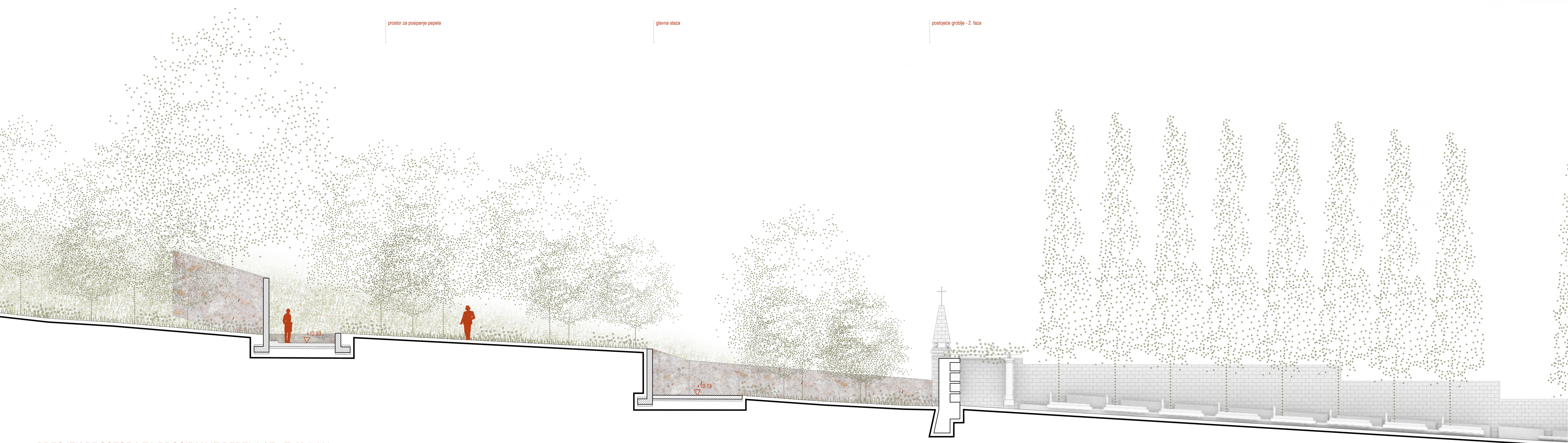
PRESJEK PROSTORA ZA PROSIPANJE PEPELA / E - E M 1:100
