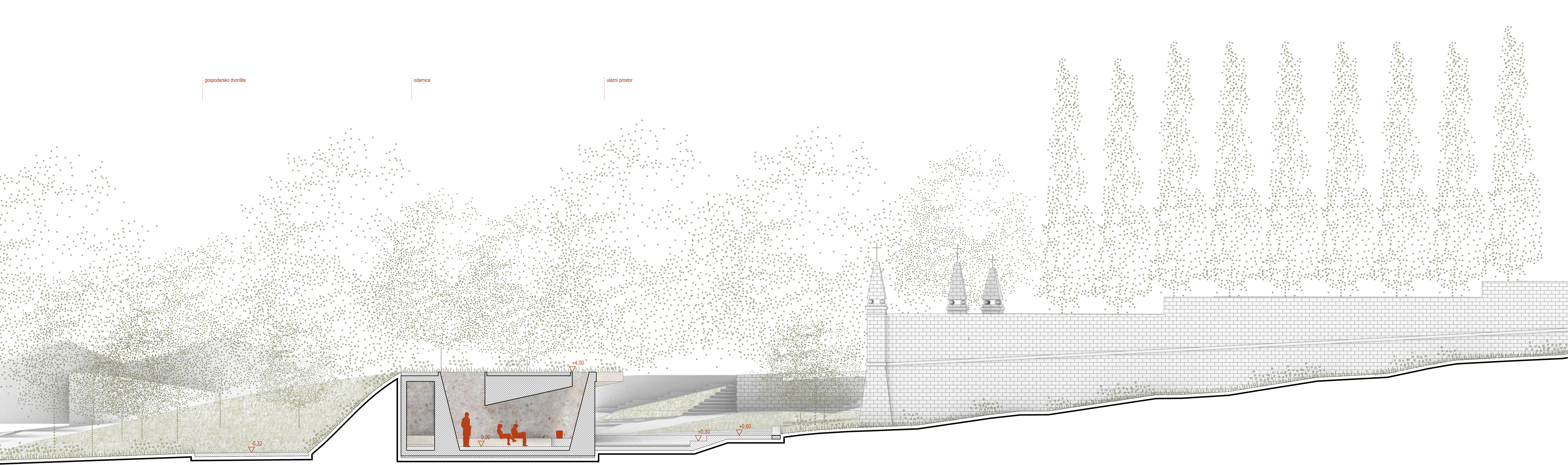
PRESJEK ODARNICE / F - F M 1:100
