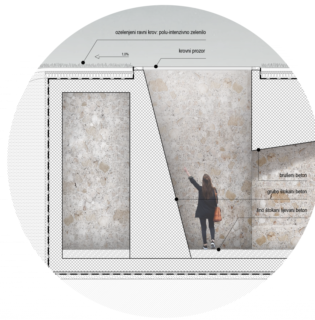
Detaji svjetlarnika v oprostajnem prostoru M 1:50
