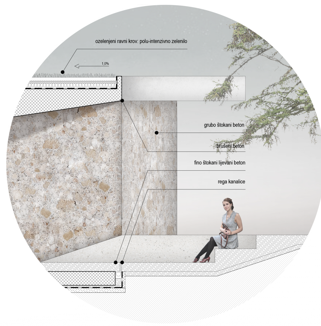
Detalj krova oprostajnog prostora M 1:50
